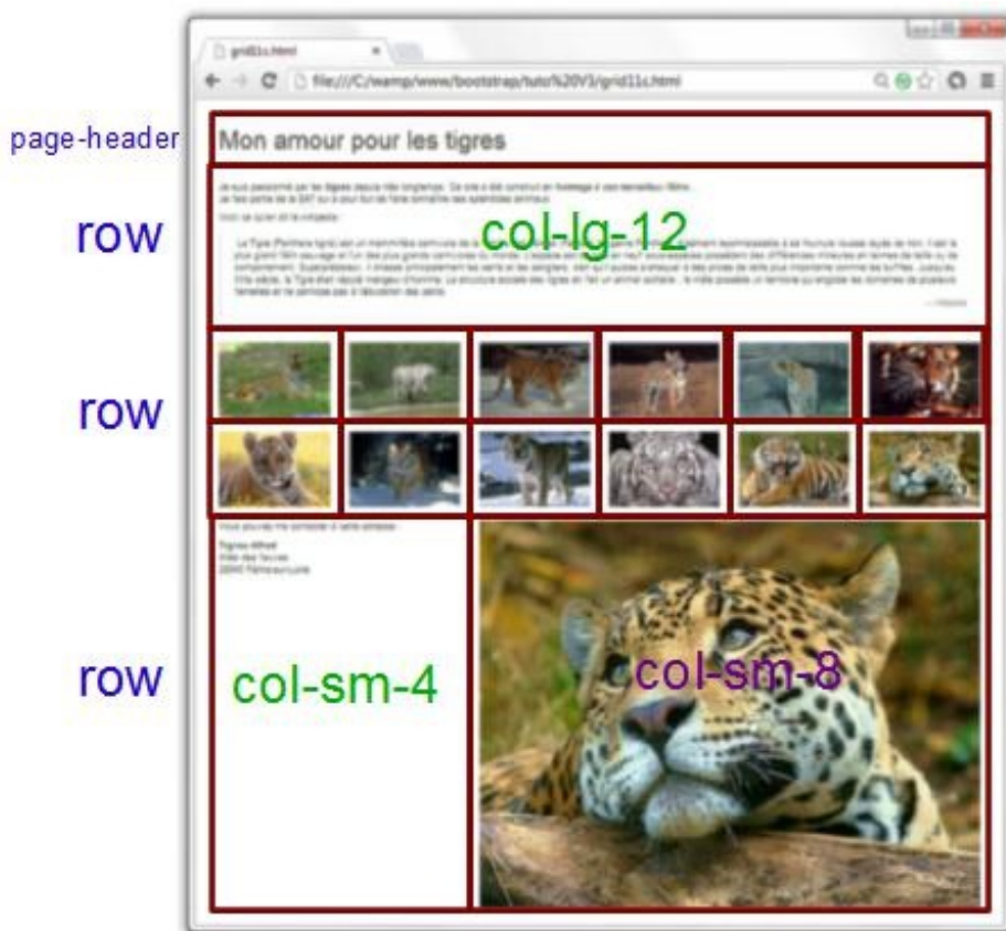
La page d'exemple décryptée
